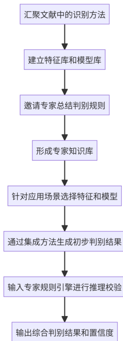
图1 机器笔迹检测系统流程
