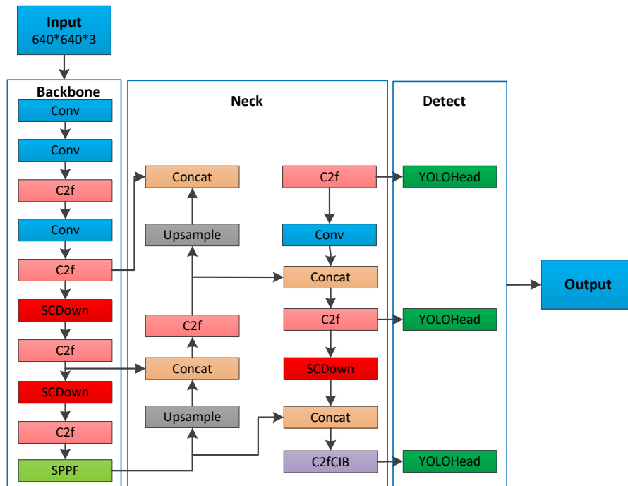
图 1 YOLOv10 网络结构
